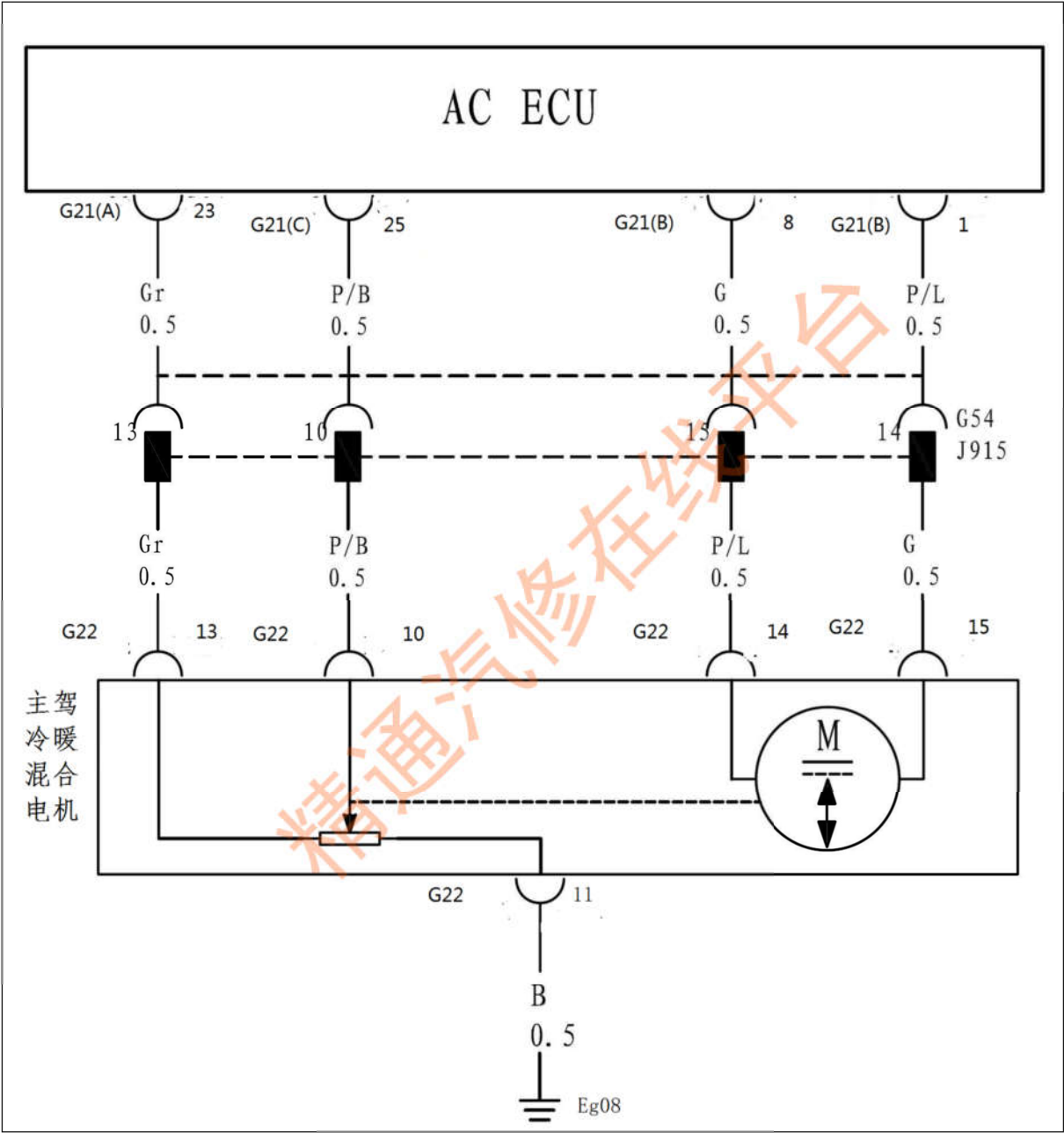
电路图
